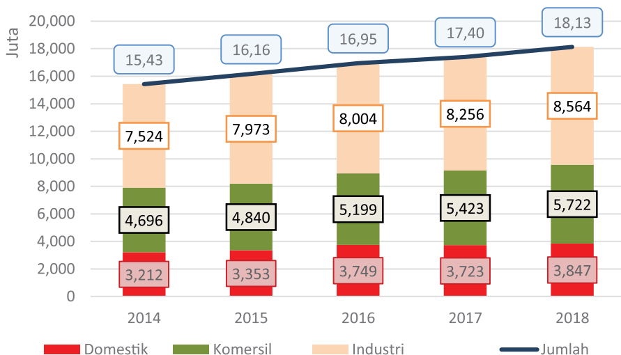
Rajah 3.4 Unit Jualan Elektrik (Juta KWJ) Mengikut Kategori Pengguna di Negeri Johor 2014-2018.
