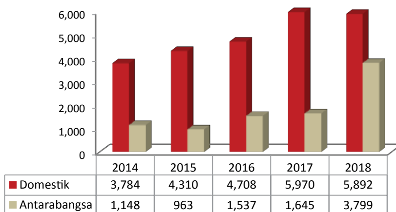
Rajah 3.19 Pergerakan Kargo di Lapangan Sultan Ismail, 2014 - 2018 ('000 tan metrik).
