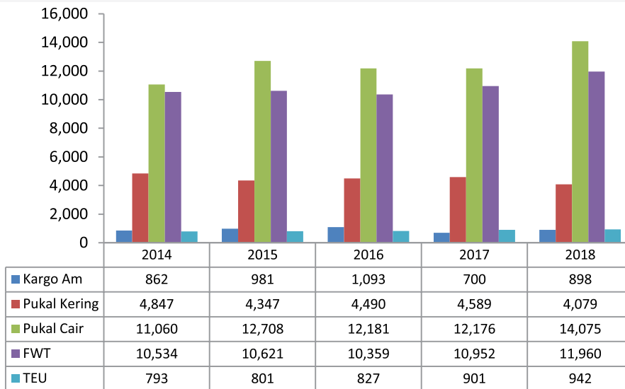
Rajah 3.17 Pengendalian Kargo dan Kontena di Pelabuhan Pasir Gudang, 2014-2017 ('000 metrik tan).
